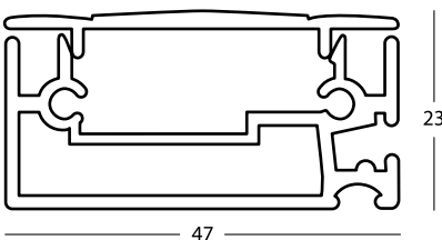
Doorsnede profiel van vaste hordeur.
